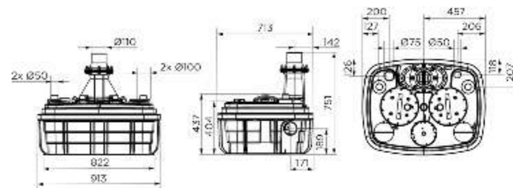
Размеры (мм)
