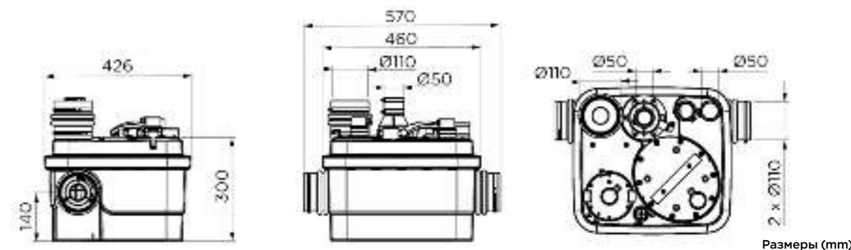
Размеры (мм)
