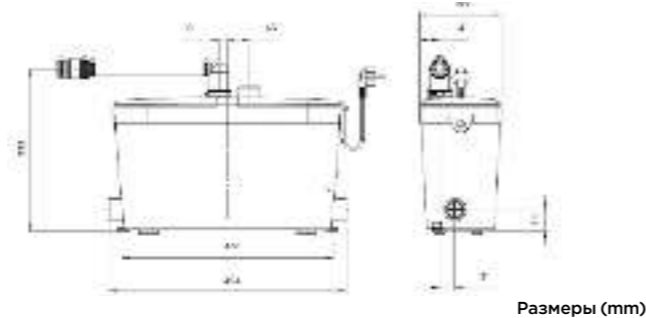
Размеры (mm)
