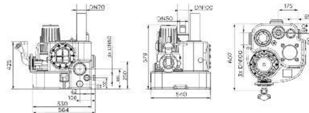
Размеры (мм)
